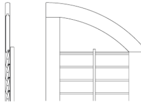
Kreisbogen Innen und Aussen
