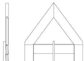
Abschrägung doppelt Innen und Aussen
